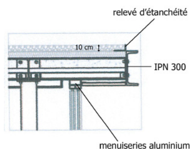
A. coupe détail du toit et des menuiseries
